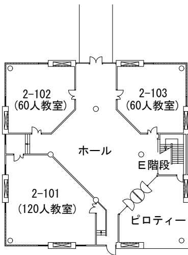
1階平面図
