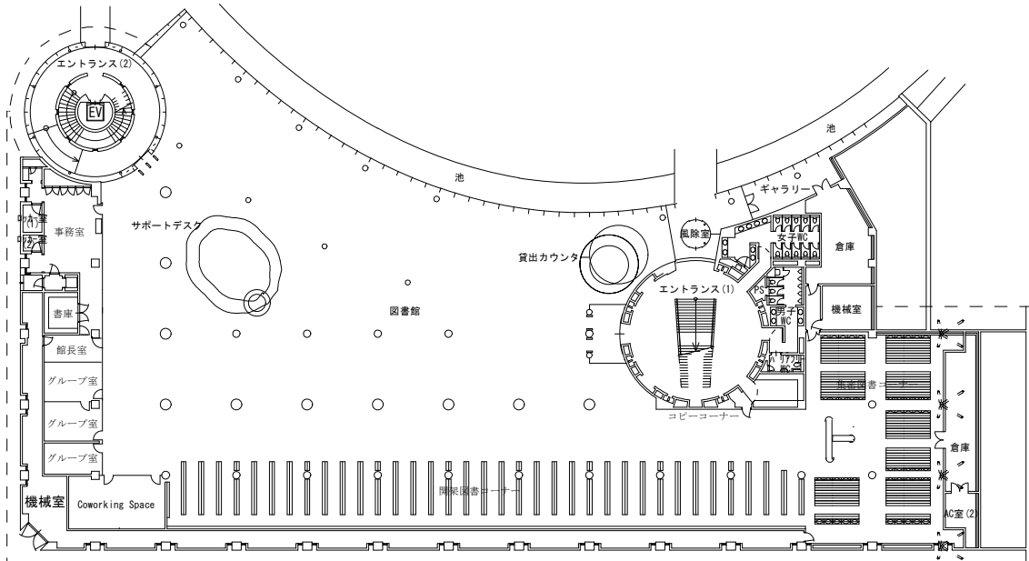
2階平面図
