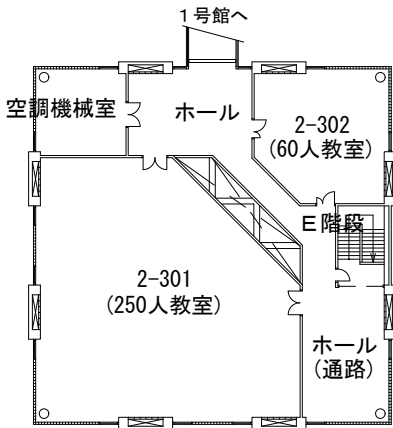
3階平面図
