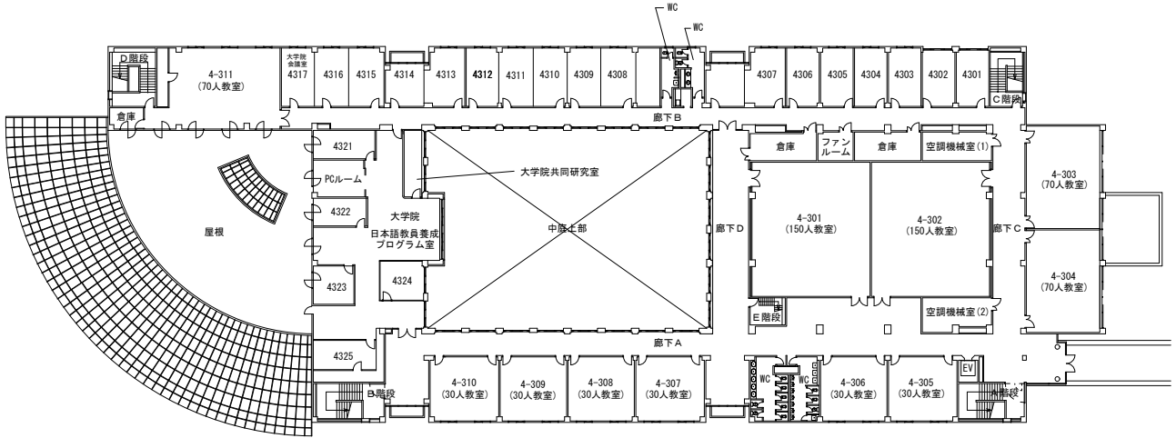
3階平面図
