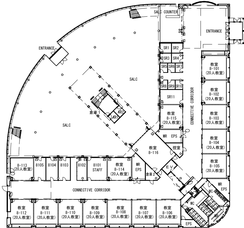
1階平面図
