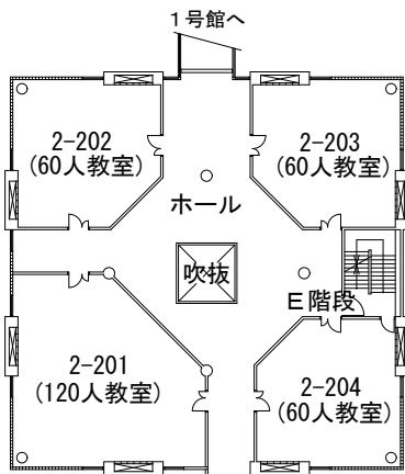
2階平面図
