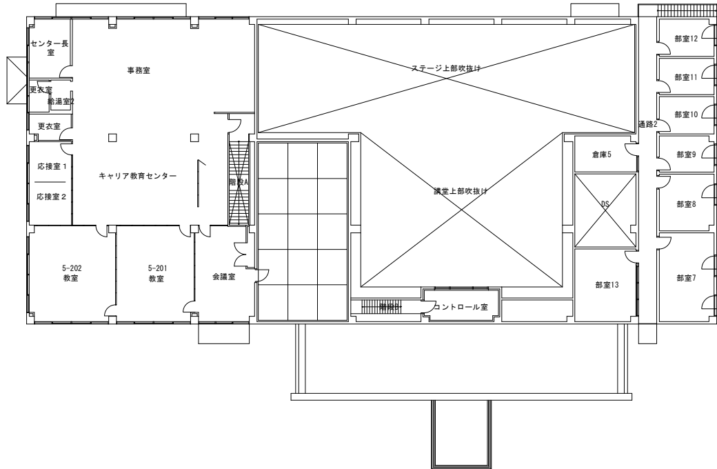
2階平面図
